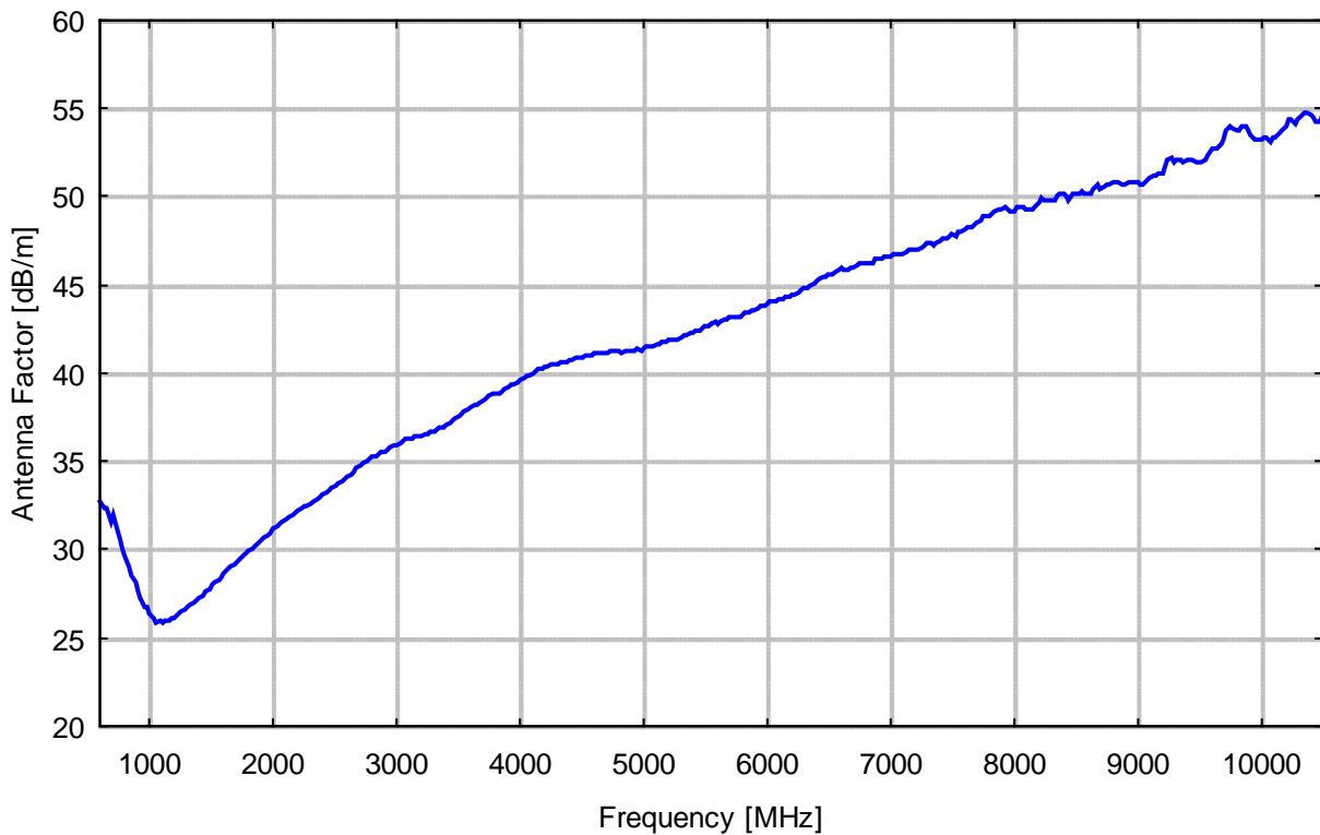
Antennen-Wandlungsmaß
